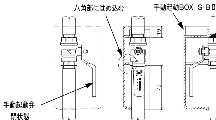
図2. 手動起動装置、取付け状態図 (手動起動BOX S-BⅡのみ断面で作図)
