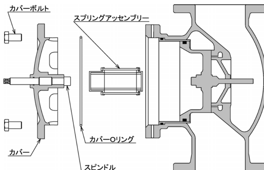
図11. カバーの取外し方法
