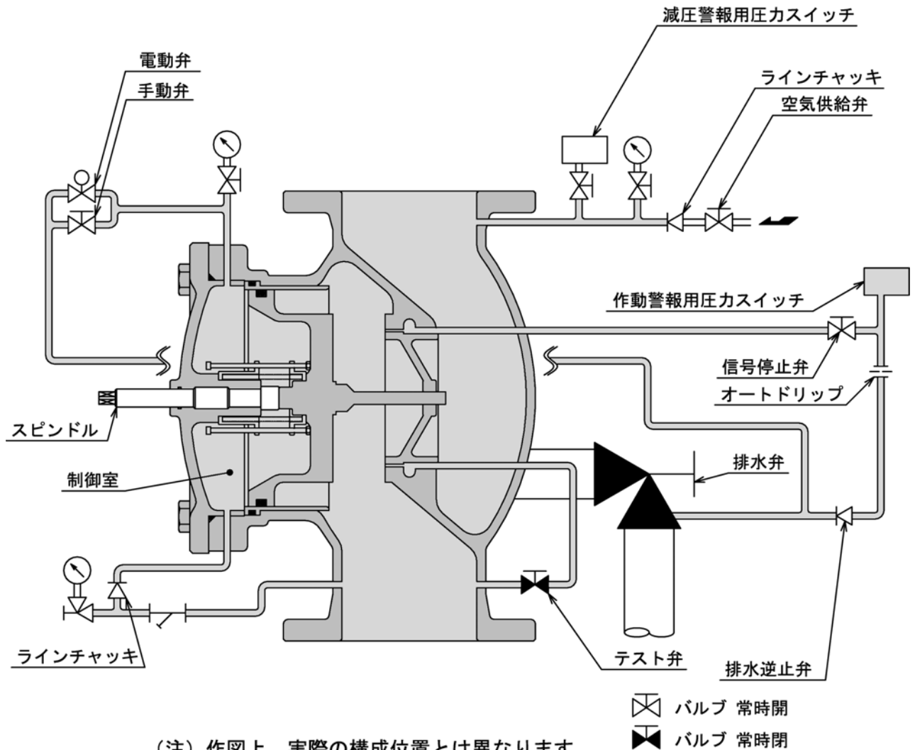
図15. 予作動式流水検知装置 ・ 作動状態
