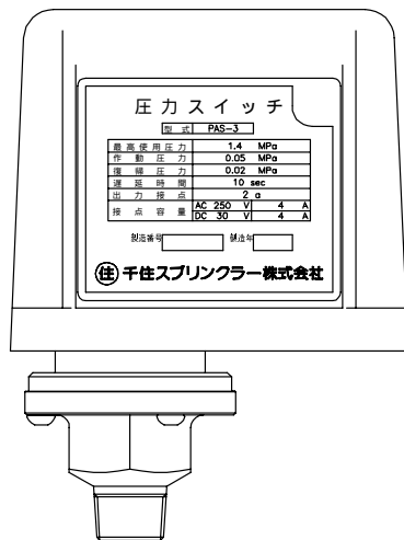
作動警報用圧力スイッチ正面図 PAS-3 型
