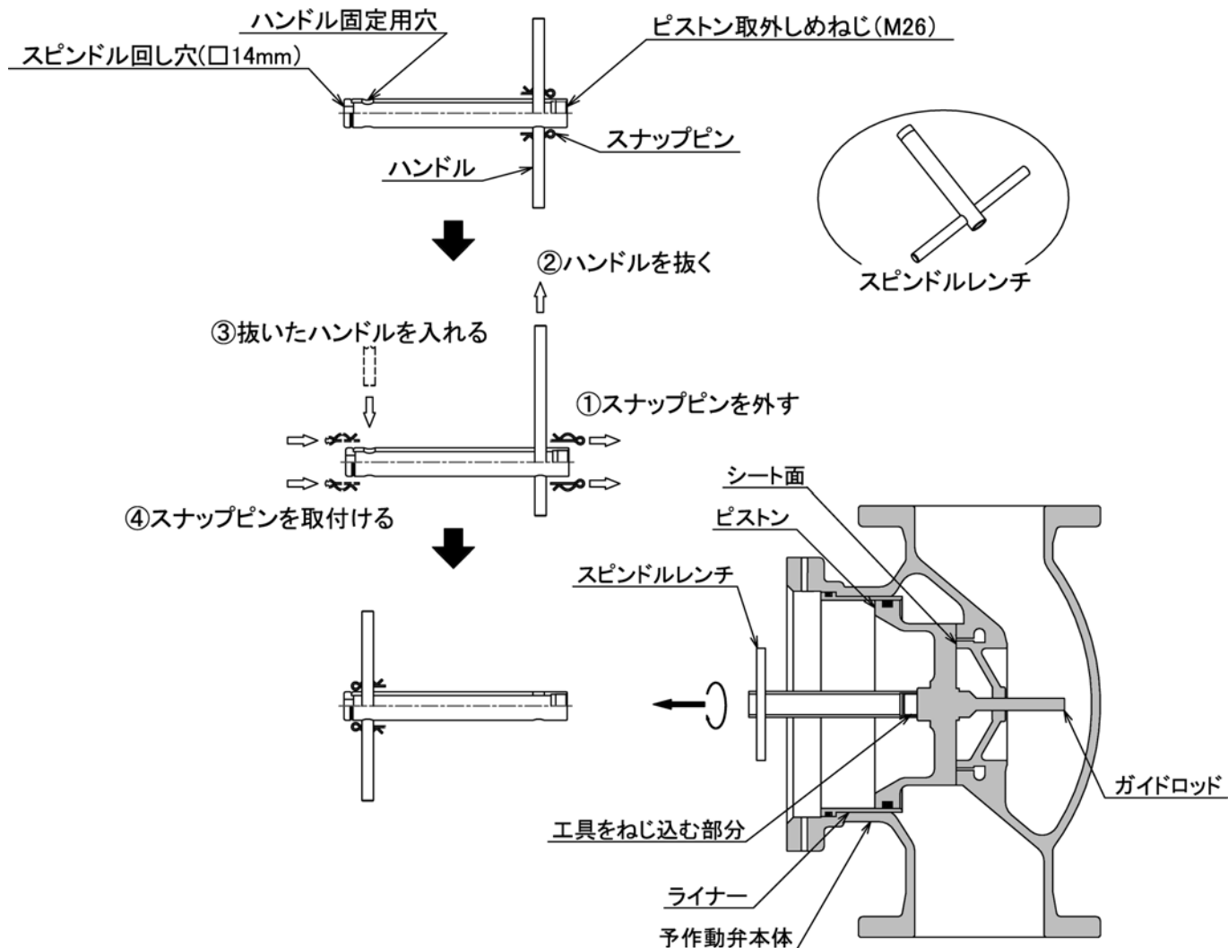
図12. ピストンの取外し方法
