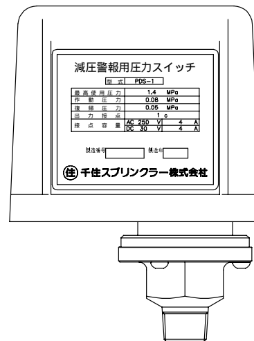
減圧警報用圧力スイッチ正面図 PDS-1 型
