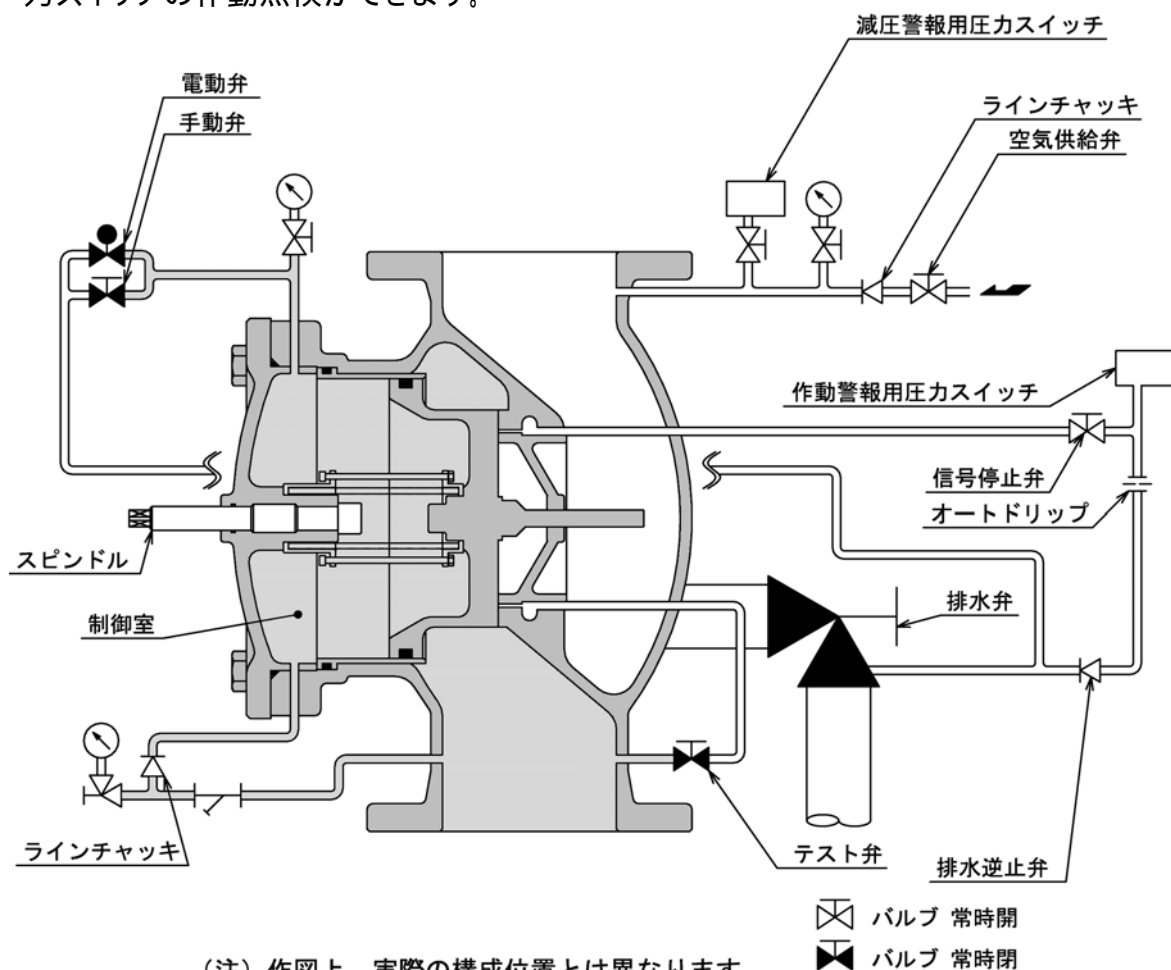
図14. 予作動式流水検知装置・警戒状態
