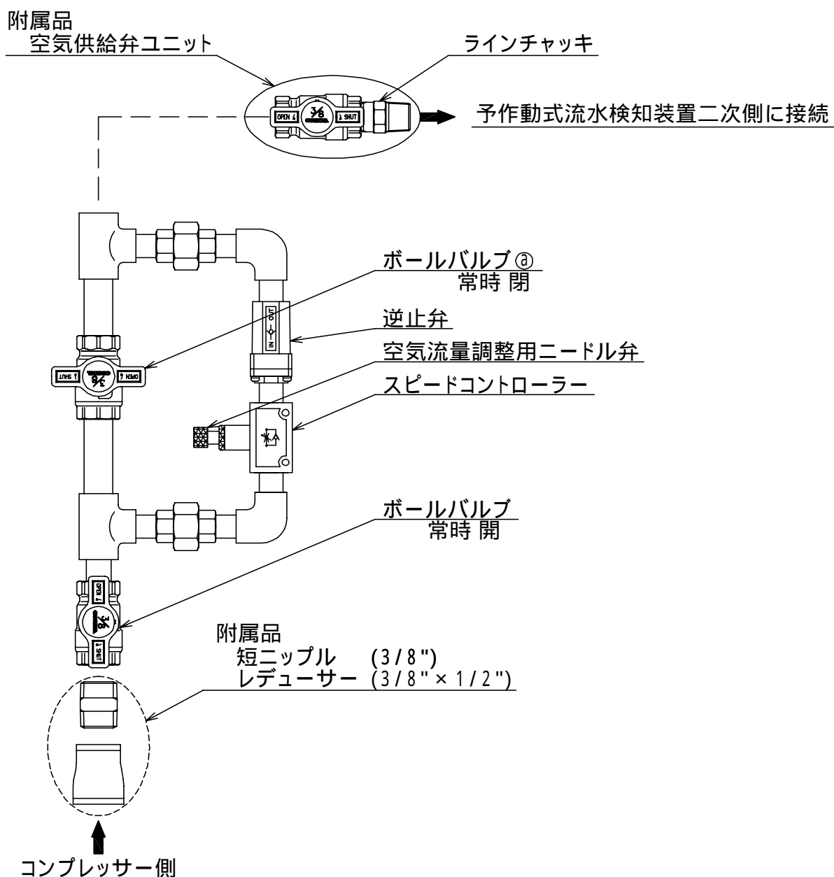
図18. スピードコントロールユニット
