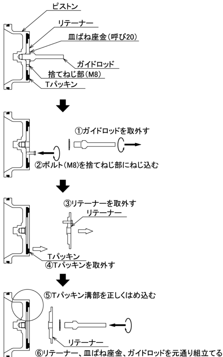
図13.Tパッキンの交換方法
