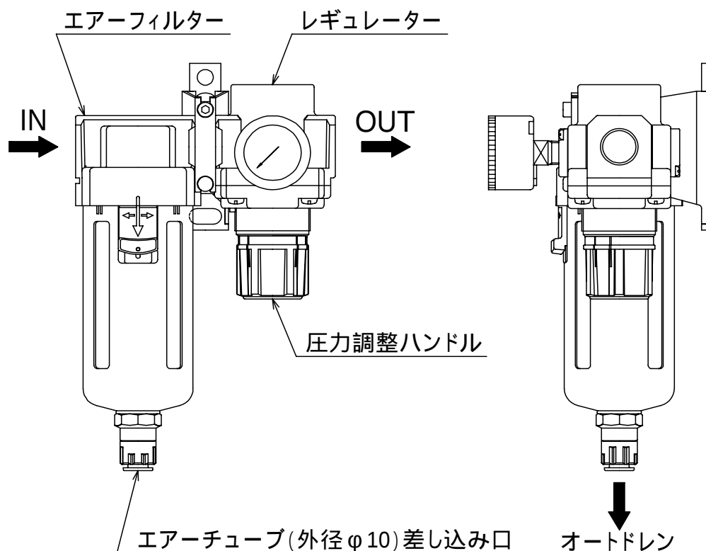
図19. レギュレーターユニット
