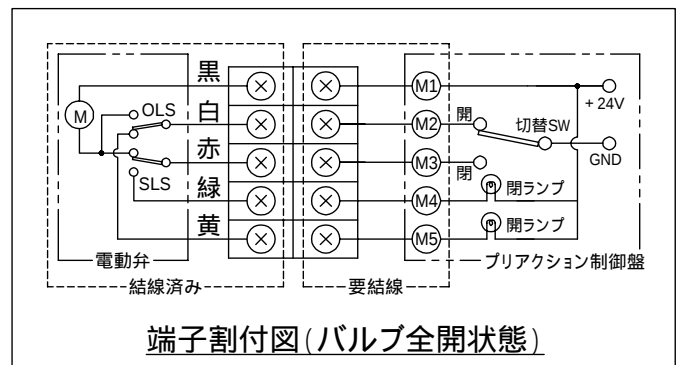
図17. 電動弁
