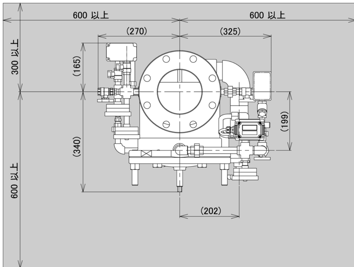
図4 . アラーム弁周囲に必要なスペース
