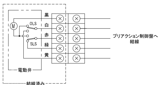
端子割付図(電動弁全閉状態)
