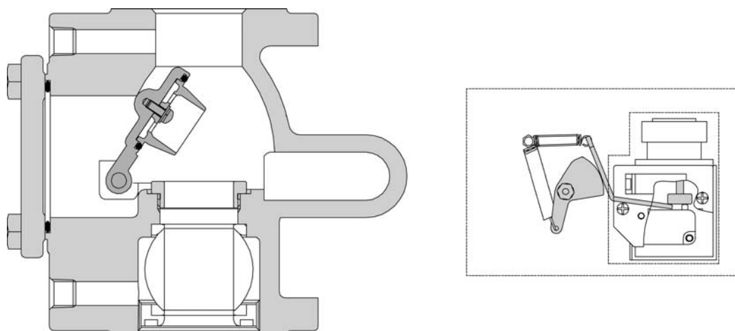
図12. CVR40U型、作動状態
