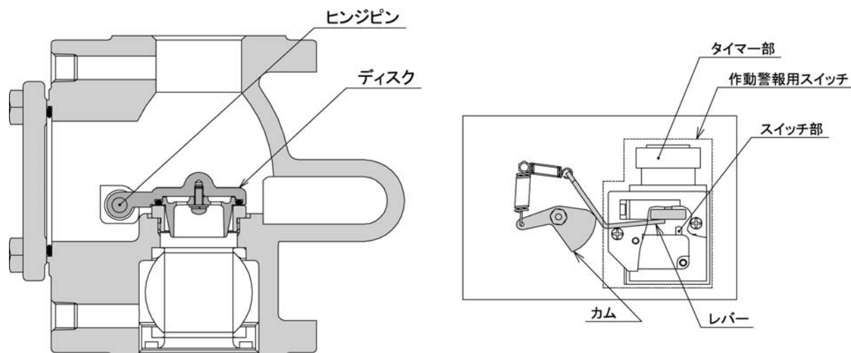
図11. CVR40U型、警戒状態
