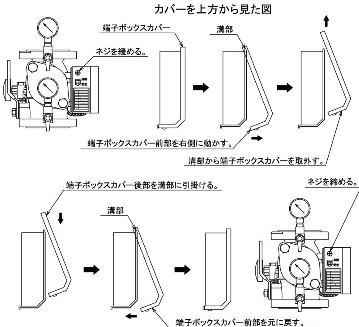
図7. カバーの脱着方法
