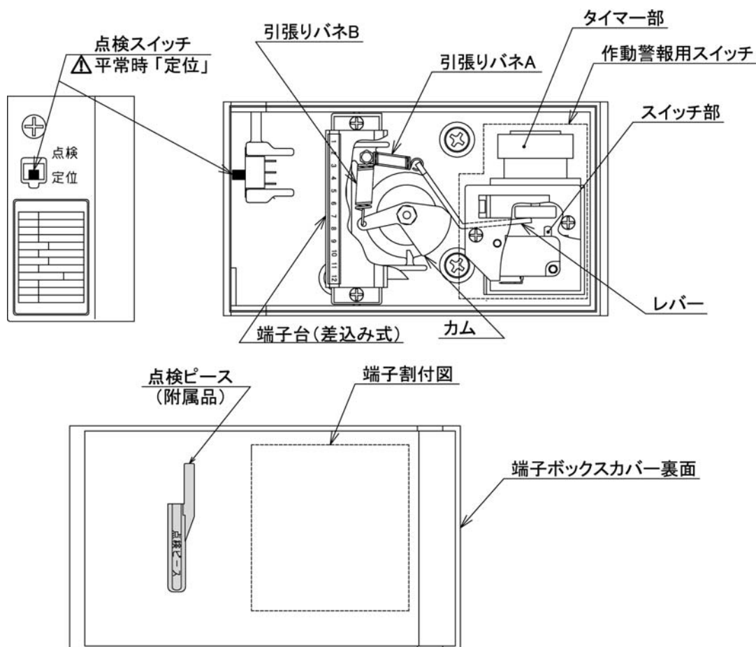
図6. 端子ボックス内部の概要図
