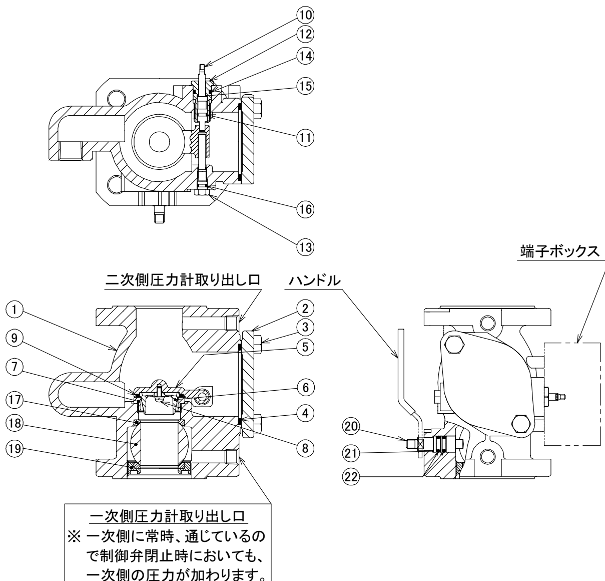
図5. CVR40U型 アラームバルブ本体
