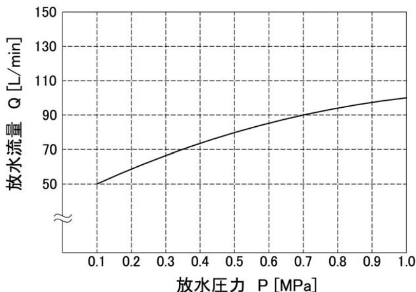
図14. 排水・試験弁 放水量特性図
