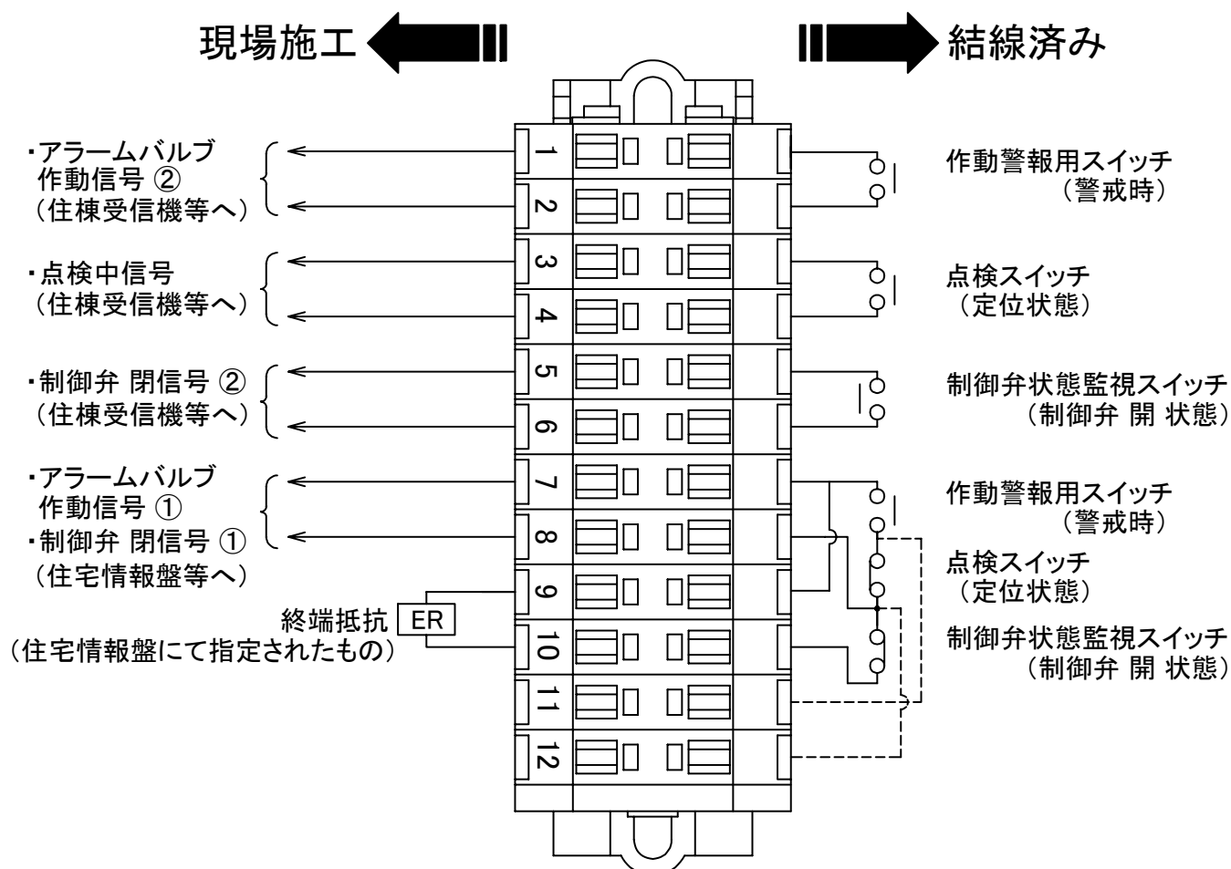
図10. 端子ボックス、結線例
