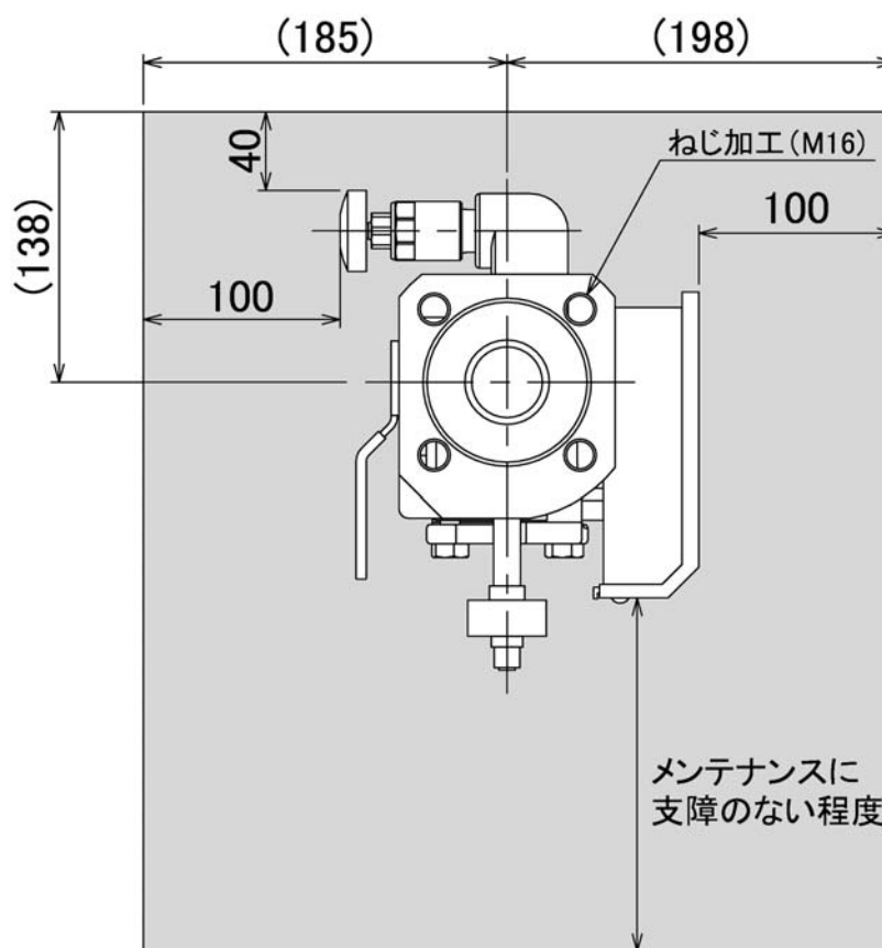
図2. アラームバルブ周辺に必要なスペース(推奨寸法)
