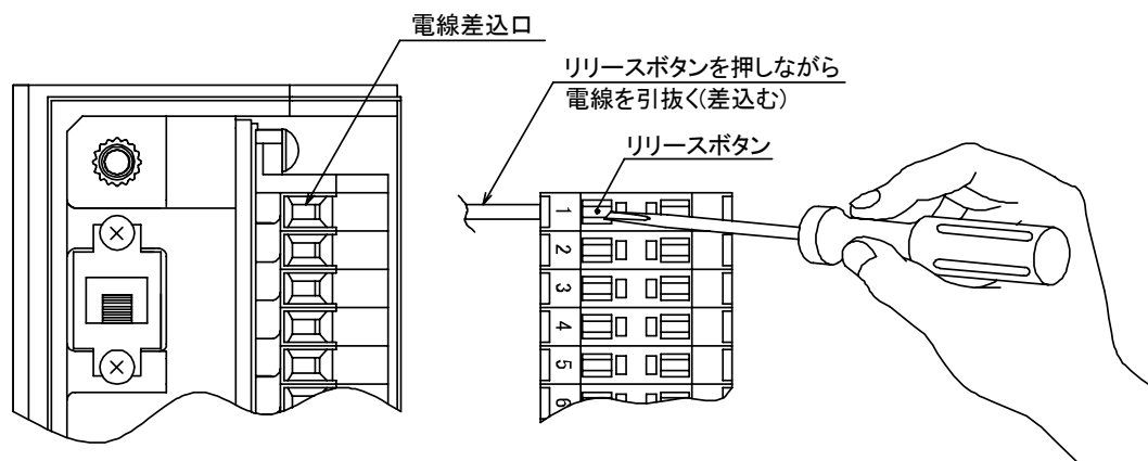
図9. 電線の引抜き、差込み方法
