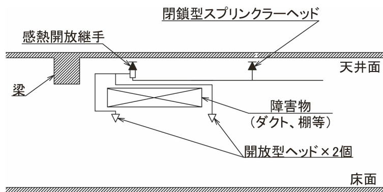
側面図
