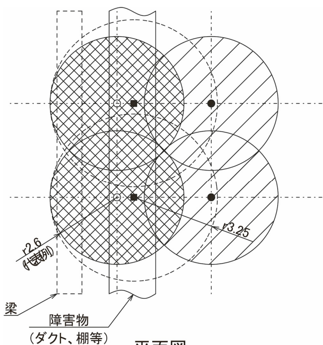
平面図
