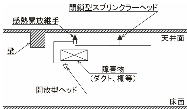
側面図
