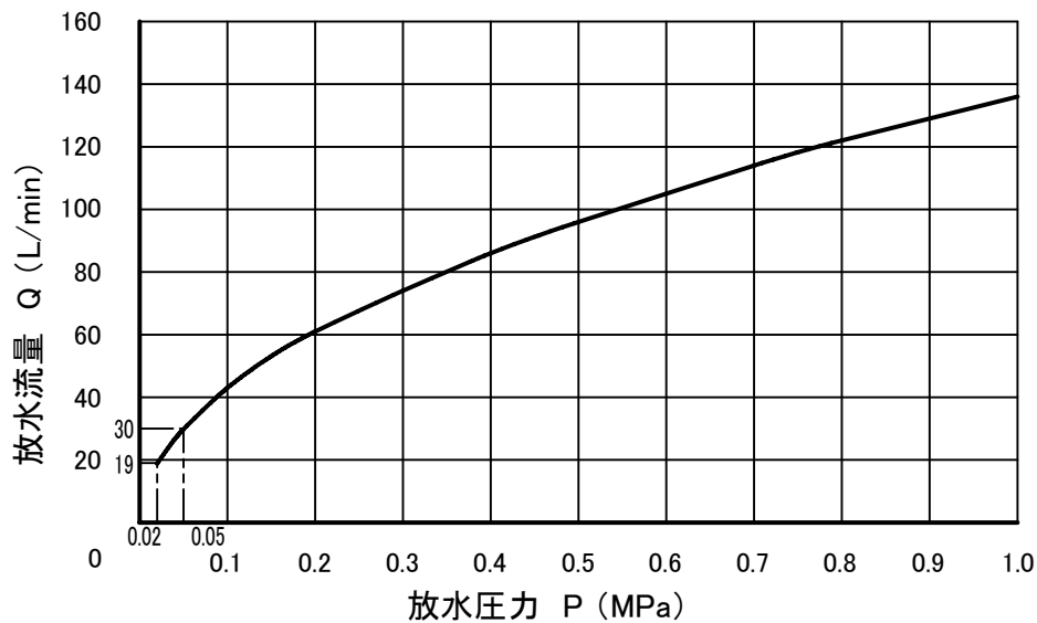
放水量特性 P-Q曲線
