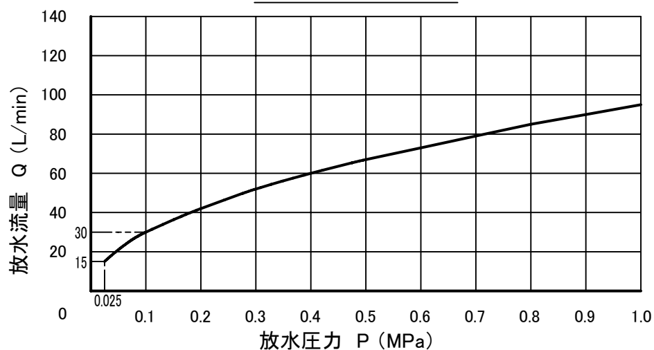
放水量特性 P-Q曲線
