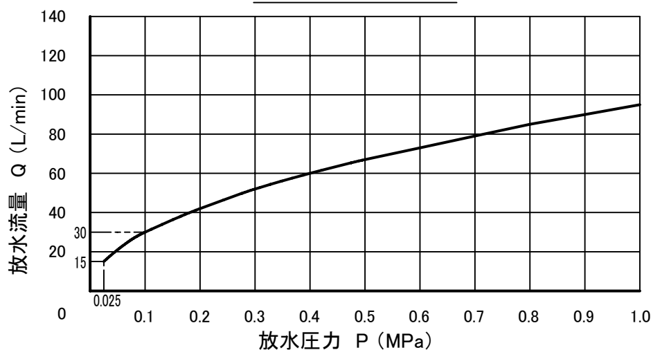
放水流量特性 P-Q 曲線
