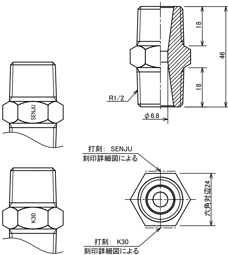
刻印詳細図
