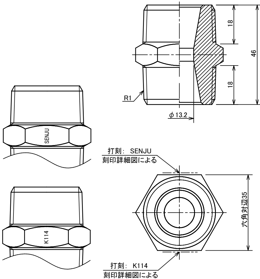
刻印詳細図
