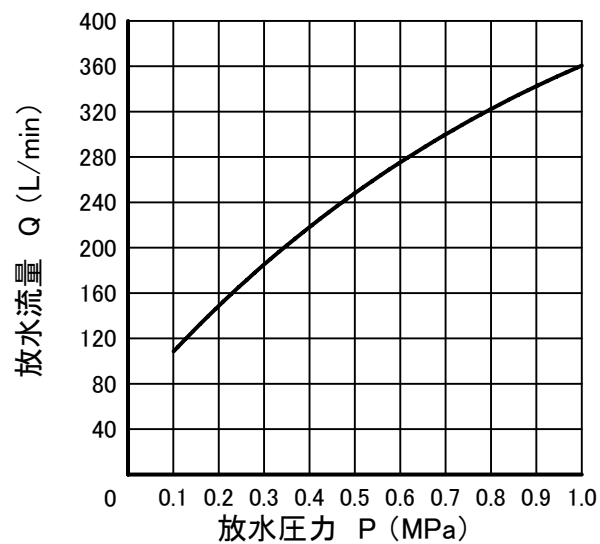
放水量特性 P-Q曲線
