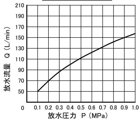
放水量特性 P-Q曲線
