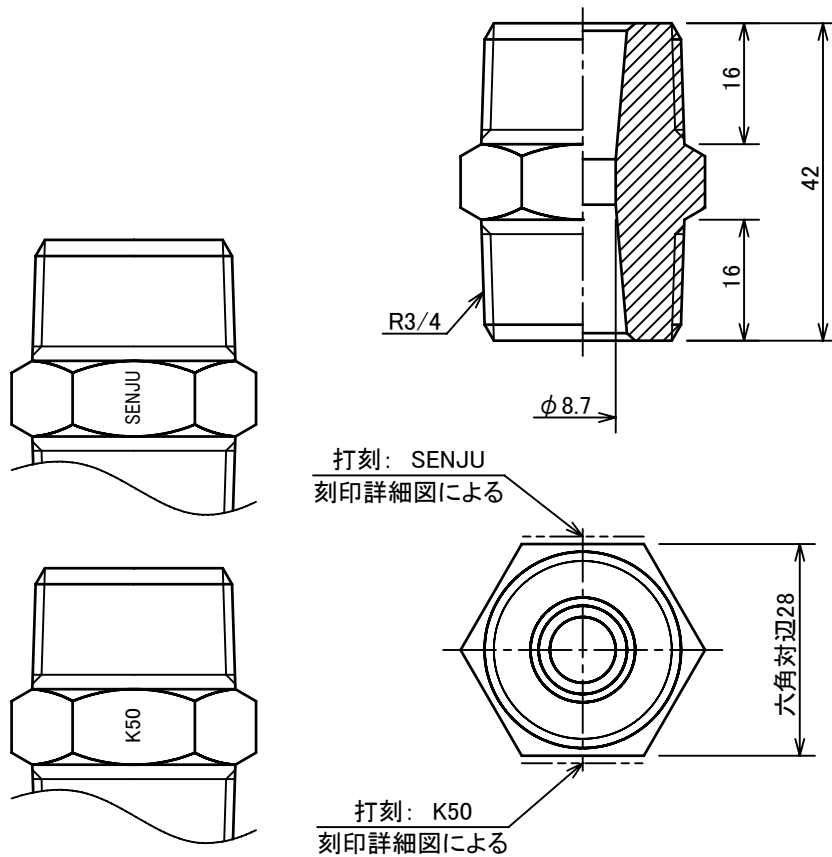
刻印詳細図
